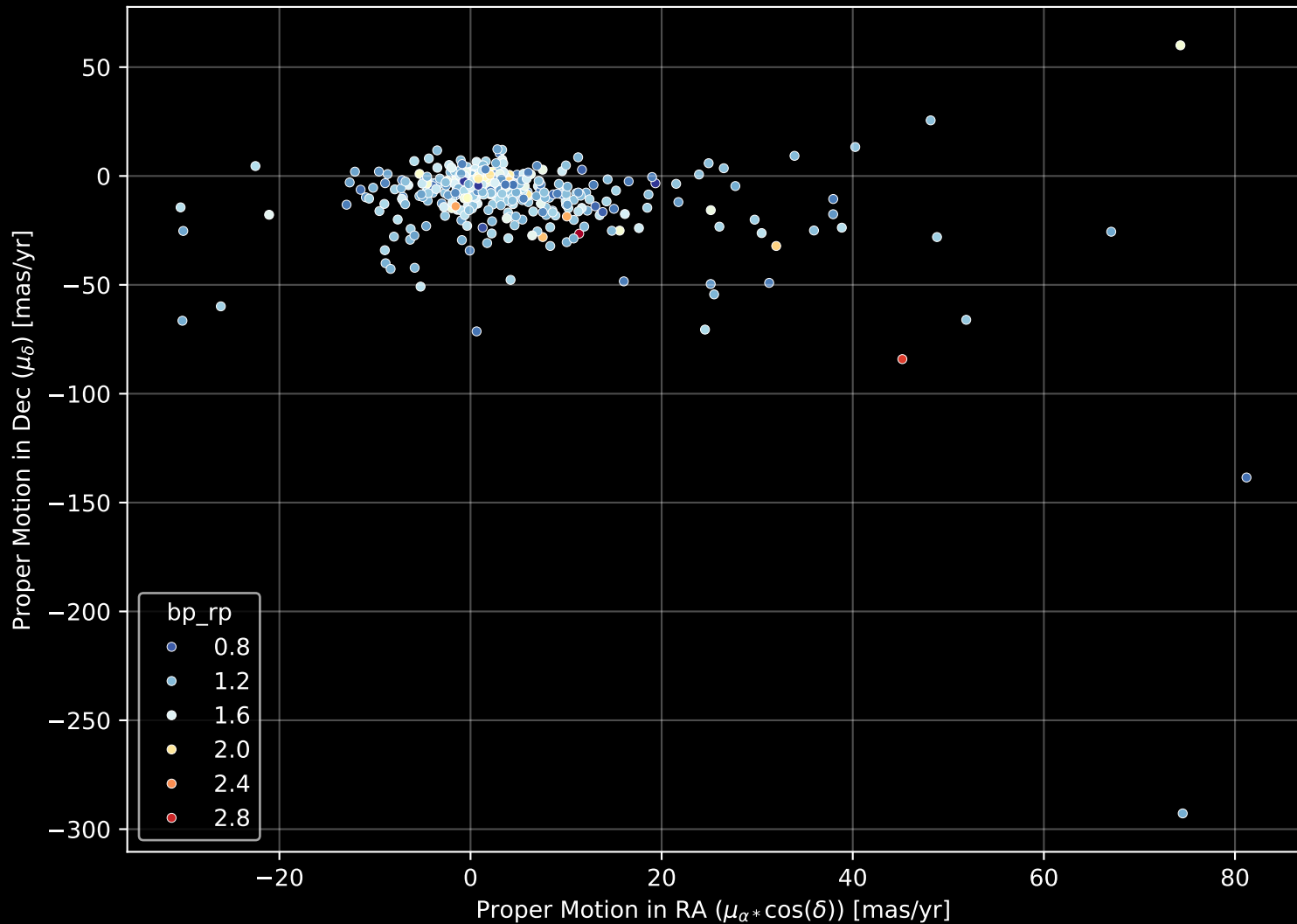
GALAH DR4 Field: [6780] Proper Motion Diagram (n= 471)
