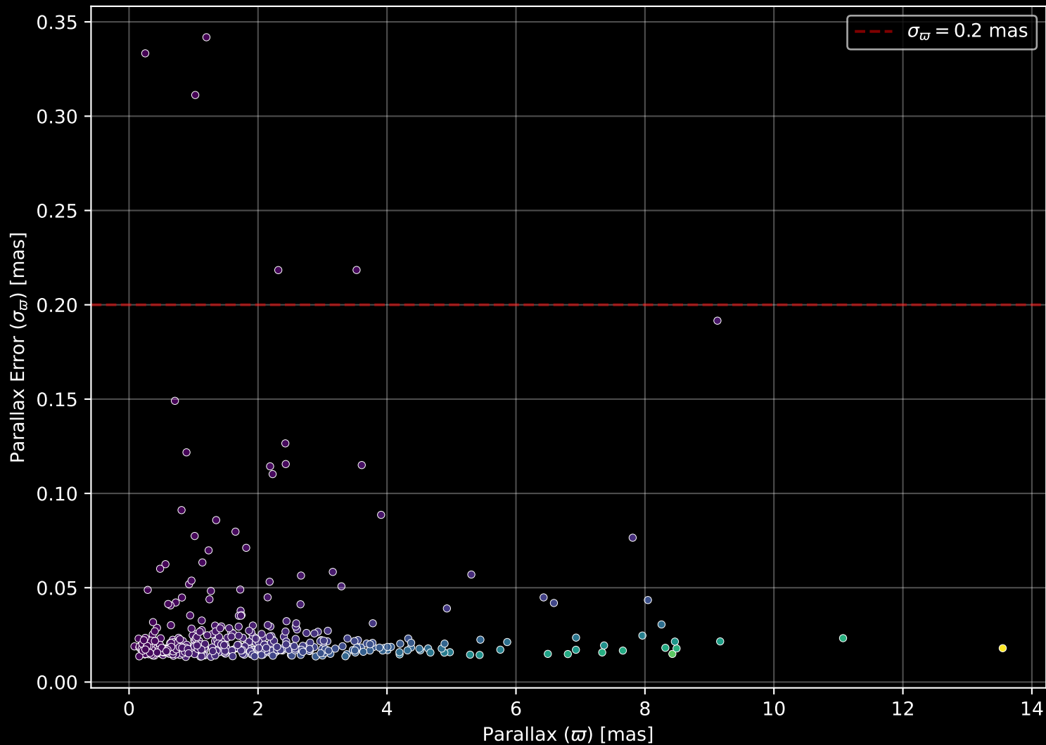
GALAH DR4 Field: [6780] Parallax Quality (n= 471)
