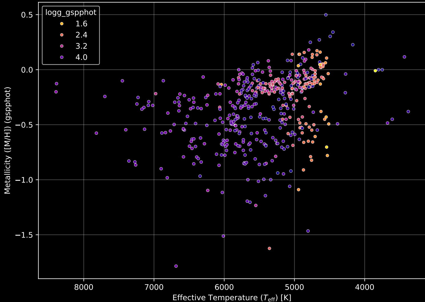
GALAH DR4 Field: [6780] Stellar Population Parameters (n= 471)
