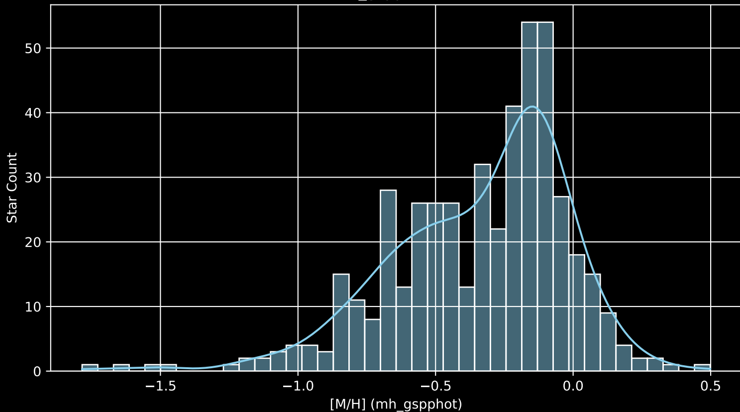
GALAH DR4 Field: [6780] [M/H] (mh_gspphot) (n= 471)
